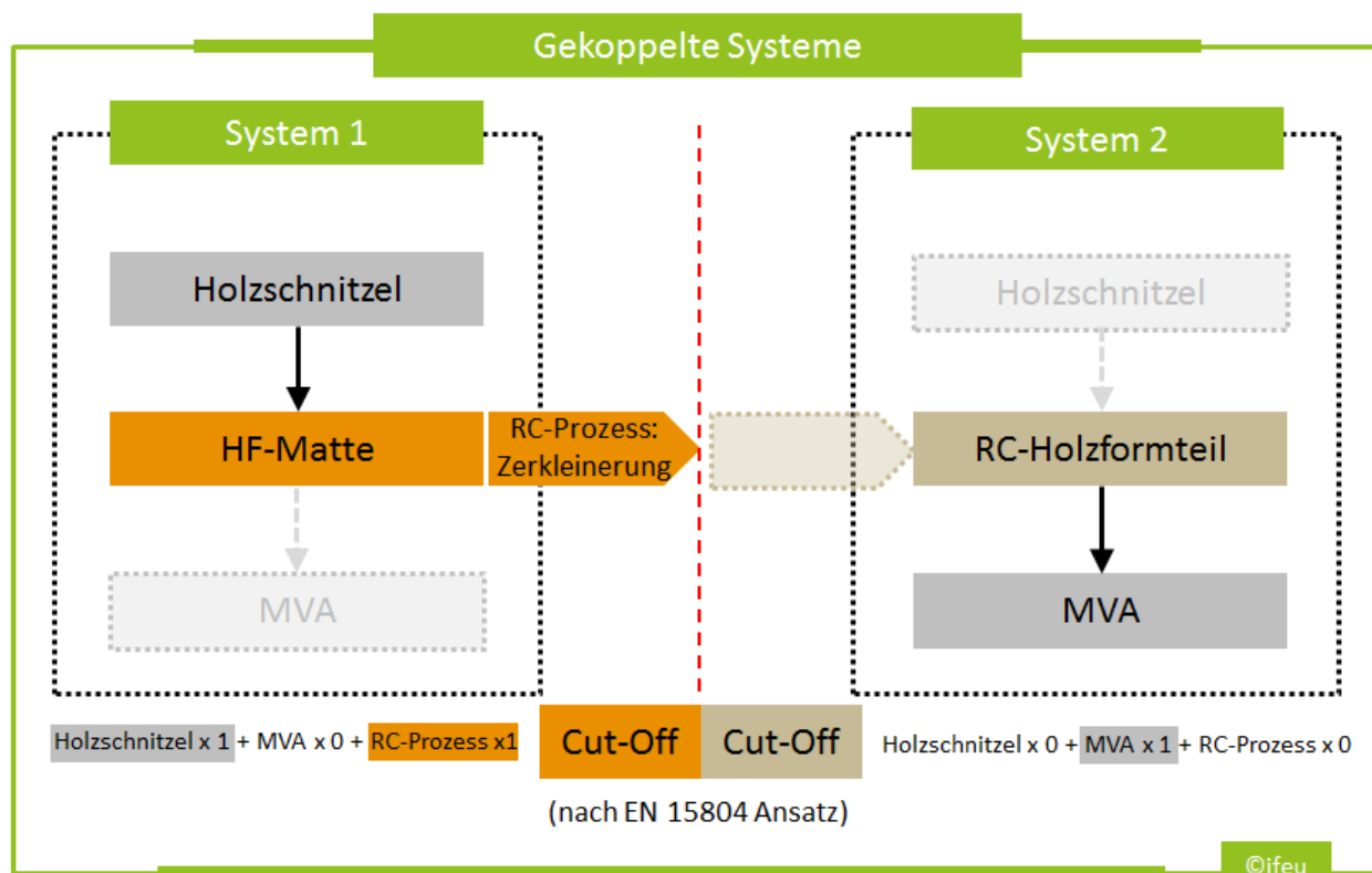
Abbildung 4-3: Kopplung der Produktion von Holzmatten (HF) über stoffliche Verwertung mit der Produktion von Holzformteilen; Aufteilung der jeweiligen Produktionslasten nach der Methodik der EN 15804 (Cut-Off-Ansatz)
