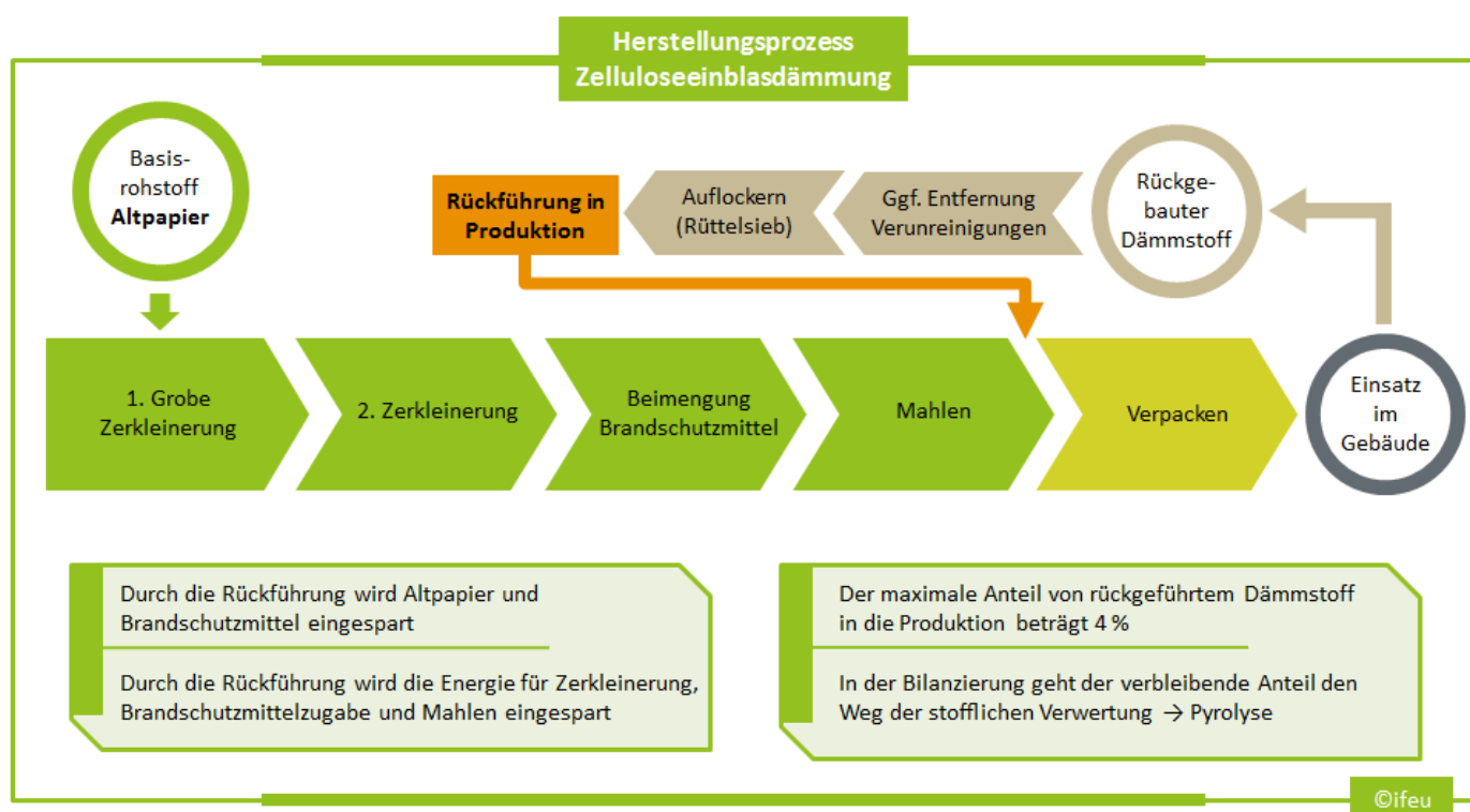
Abbildung 3-4: Vereinfachte Darstellung des Herstellungsprozesses von Zelluloseeinblasdämmung unter Berücksichtigung einer Prozessrückführung von rückgebaute Zelluloseeinblasdämmung
